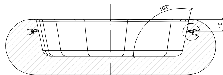
SECCIÓN / SECTION
